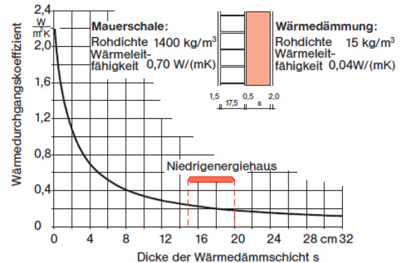
1-6 Wärmedurchgangskoeffizient U einer einschaligen Wand mit Wärmedämm-Verbundsystem
